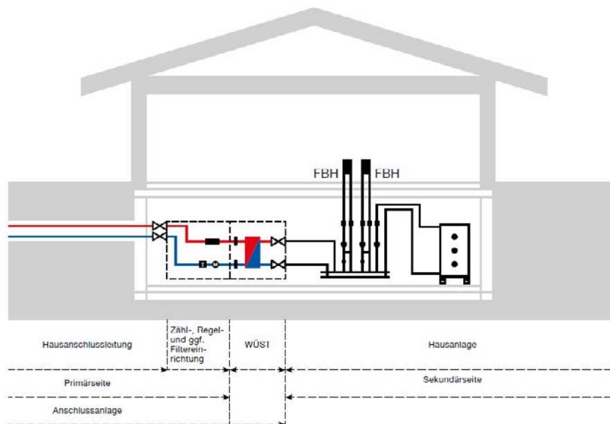
Abbildung 1: Grenze zwischen Hausanschlussleitung, WÜST und Hausanlage
