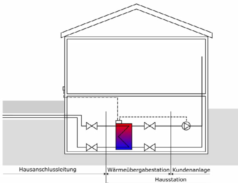
Abbildung 1: Grenze zwischen Hausanschlussleitung, Wärmeübergabestation und Hausanlage
